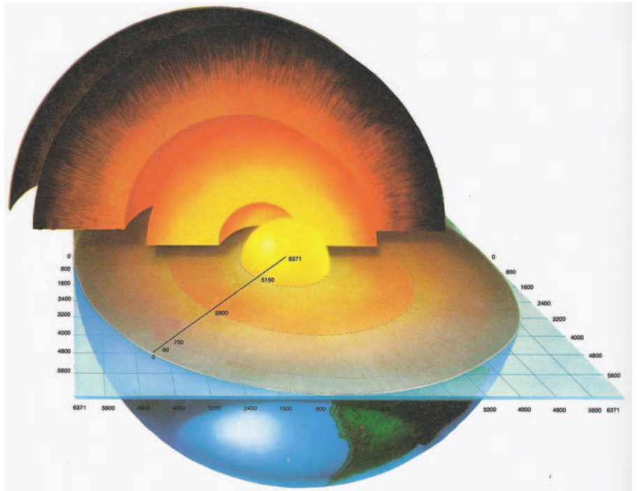
Schalenaufbau der Erde - Zahlenangaben in km.
