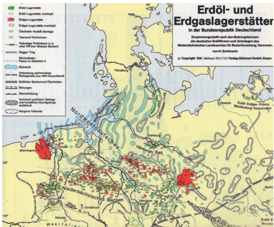
Erdöl- und Erdgaslagerstätten in der Bundesrepublik Deutschland
